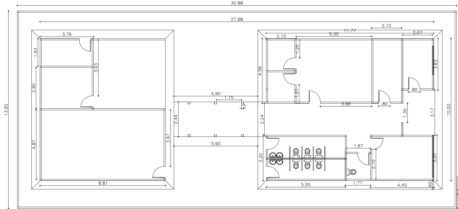
01 PLANTA BAIXA ESCOLA MUNICIPAL OTILHA ESCALA
