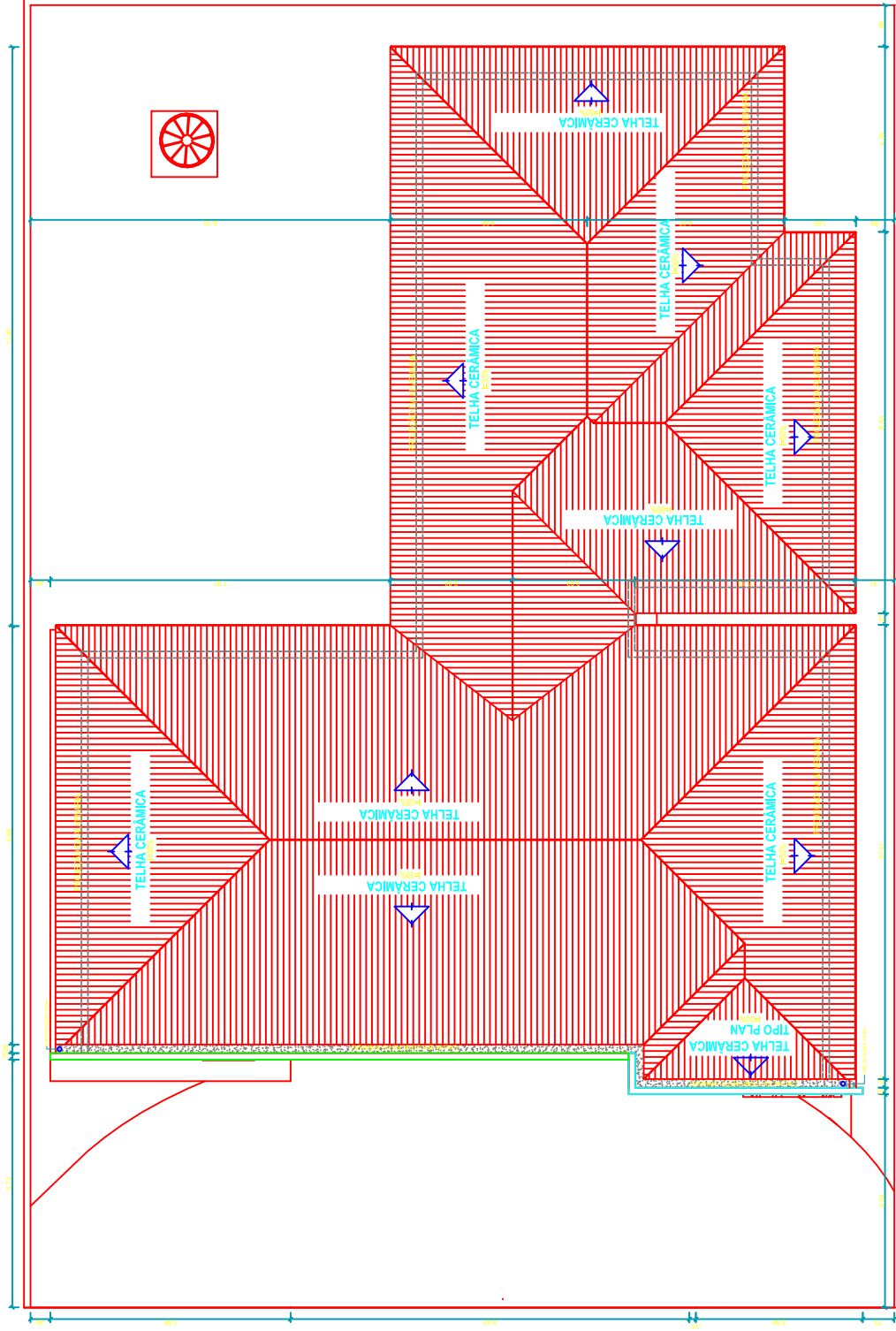
03 PLANTA BAIXA COBERTURA 48cm x 18m
