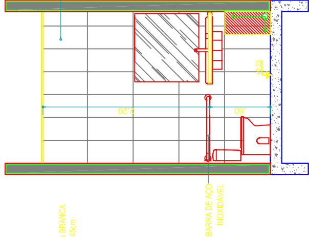
28 BHO PNE F.- CORTE 04 ESC.: 1:35
