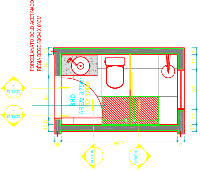
34 BHO FUNCIONÁRIOS- VISTA SUPERIOR ESC.: 1:35
