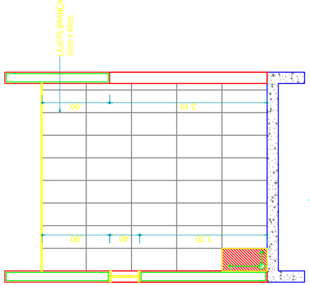
37 BHO FUNCIONÁRIOS- CORTE 03 ESC.: 1:35
